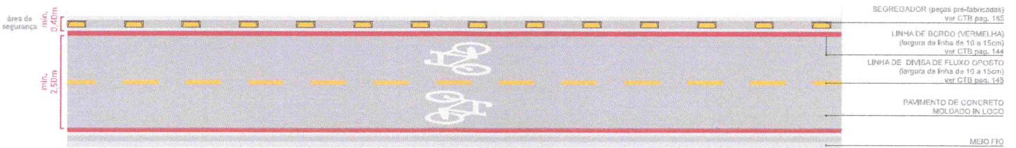
PLANTA - CICLOVIA BIDIRECIONAL
