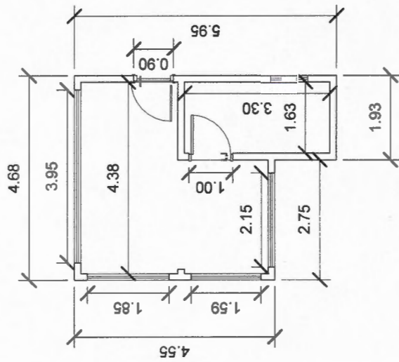
2. PAV. TERREO
