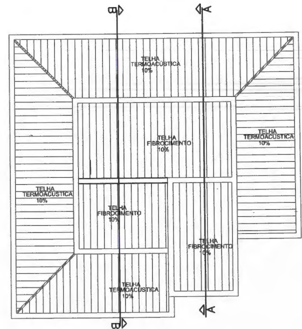
PLANTA COBERTURA ESC 1:50
